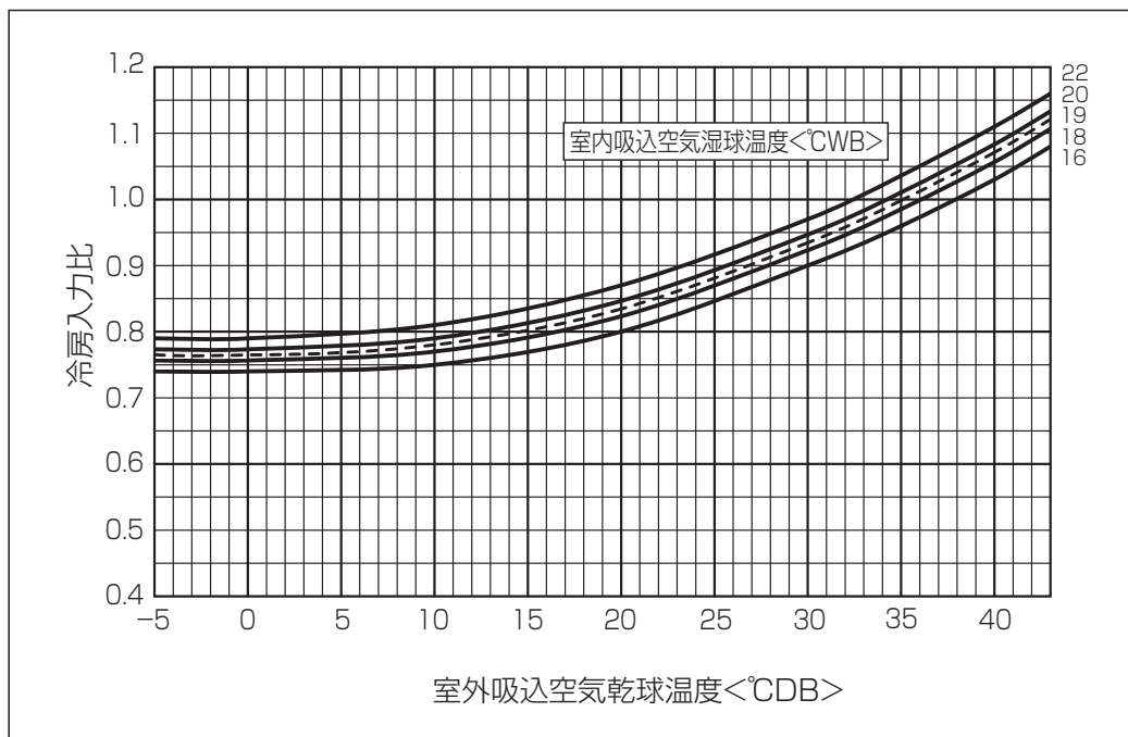
■冷房入力線図 PUZ-ZRP・KA7/HA13, PUZ-ERP・KA7/HA13/LA2, PU-CRP・KA7/HA13/LA2
