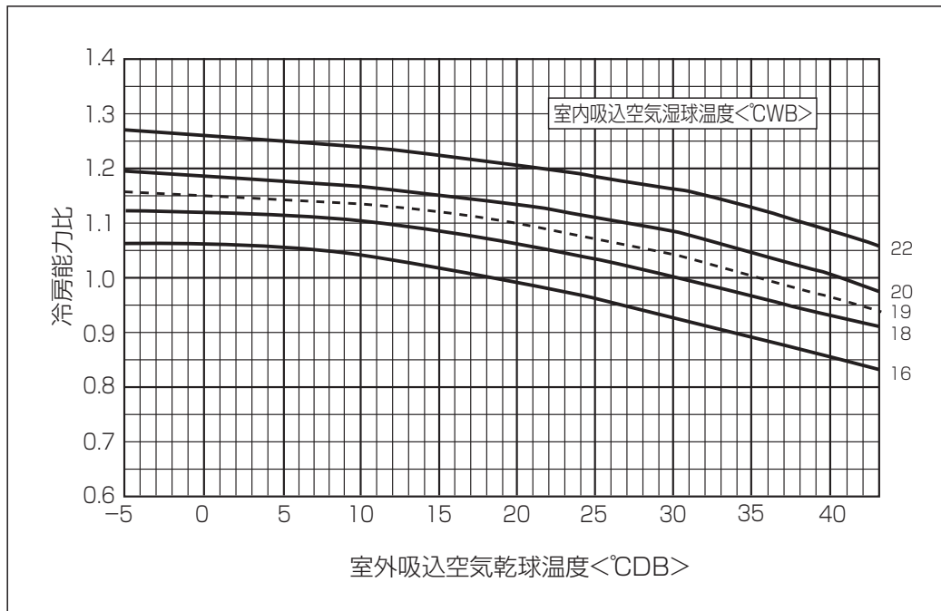
■冷房能力線図 PUZ-ZRP・KA7/HA13, PUZ-ERP・KA7/HA13/LA2, PU-CRP・KA7/HA13/LA2
