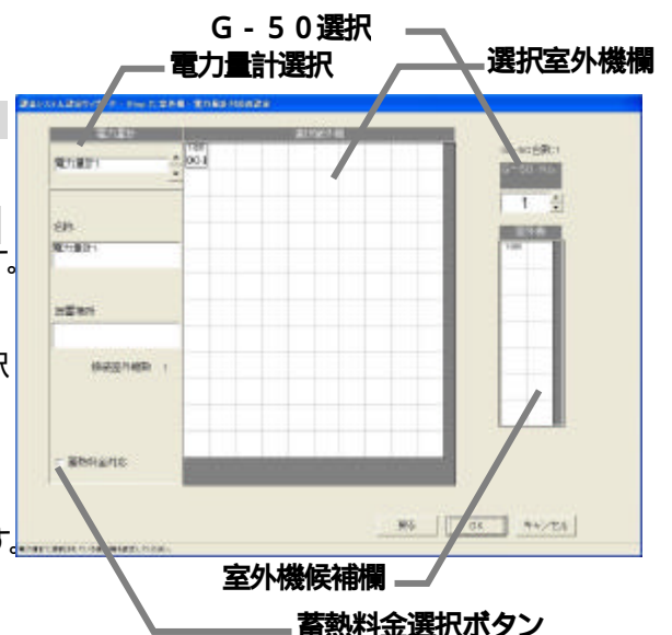
室外機 - 電力量計対応設定の画面
