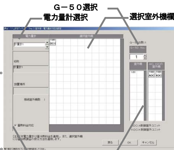
室外機候補欄 蓄熱料金選択ボタン 室外機—電力量計対応設定の画面
