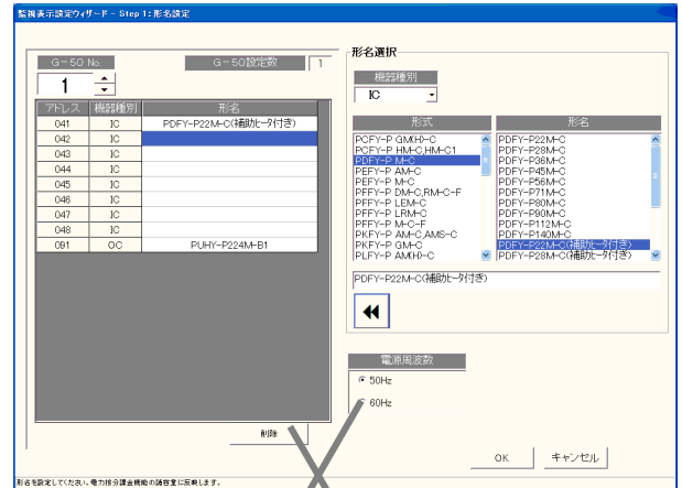
電源周波数選択 形名削除ボタン
