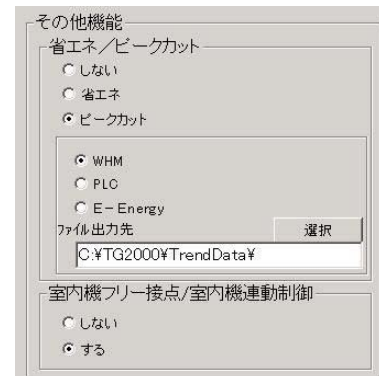
その他②の機能設定画面
