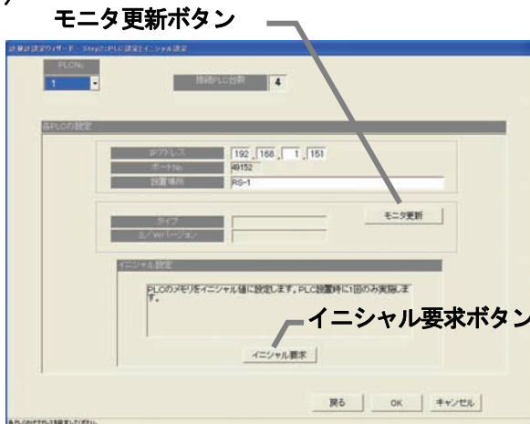
PLC接続設定画面
