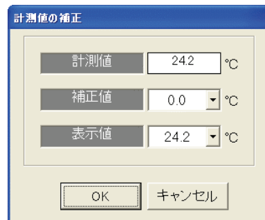
計測値の補正画面
