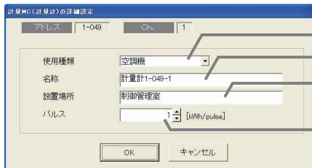
計量計詳細設定画面
