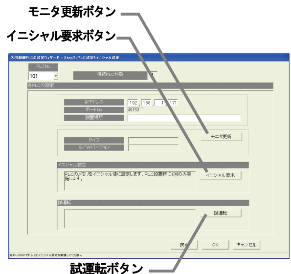
PLC接続設定画面
