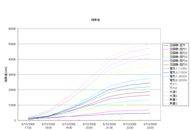
電力量計のトレンドグラフ例
