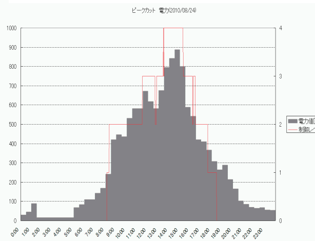
ピークカット日報(電力)のトレンドグラフ例
