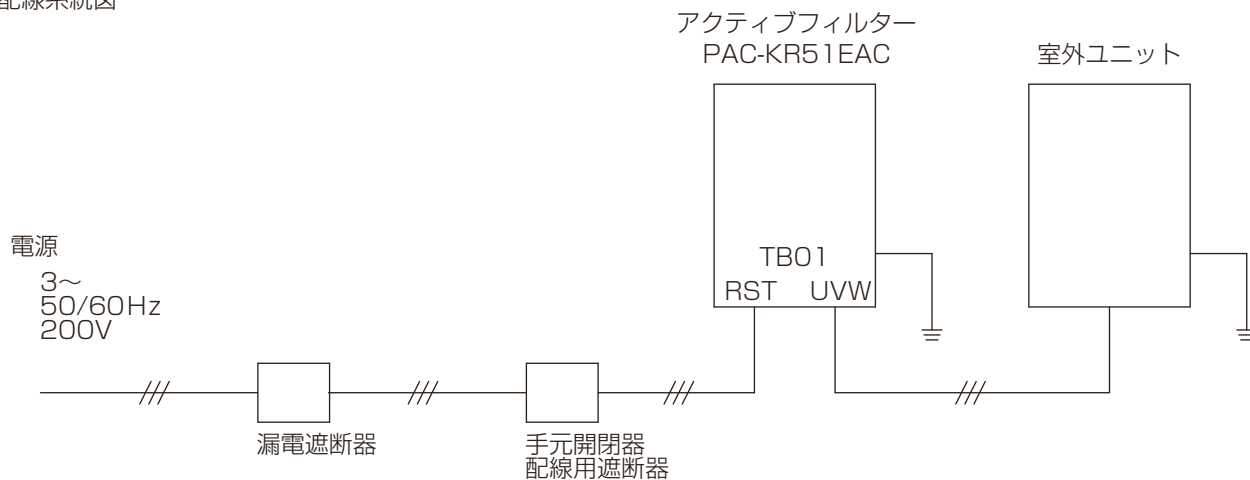
配線系統図
