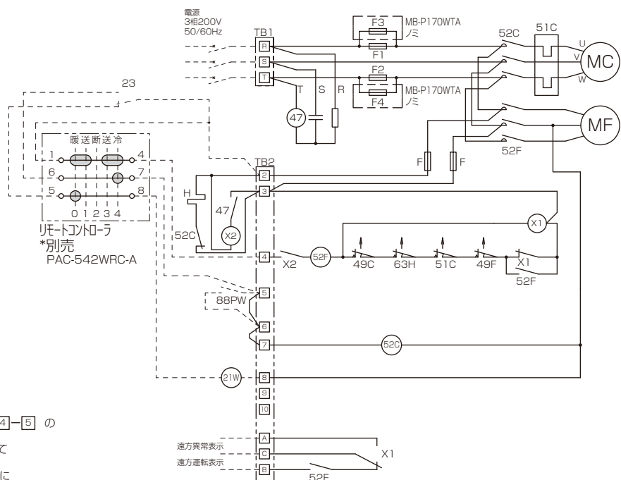
MB-P100WTA,170WTA 電気回路図
