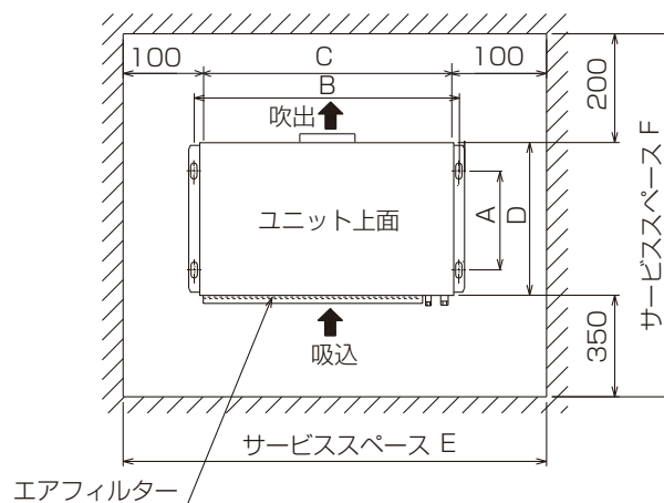
(図2) MB-P100,P170WTA/MTAの場合
