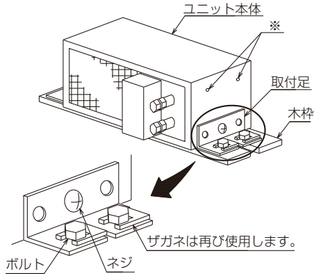
(図3-A) WT形の場合
