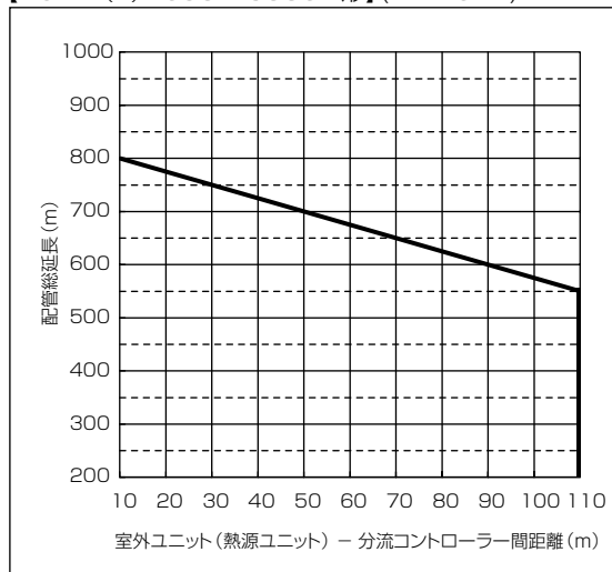
【PURY-(E)P690/730SCM形】(24/26HP)
