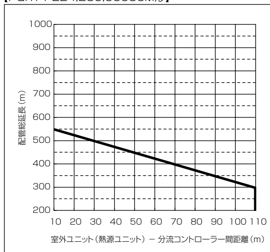
【PURY-P224,280,335SCM形】
