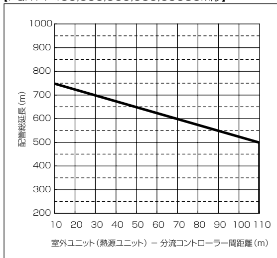
【PQRY-P450,500,560,630,690SCM形】
