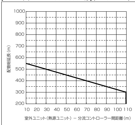
【PURY-(E)P224/280/335CM形】(8/10/12HP)
