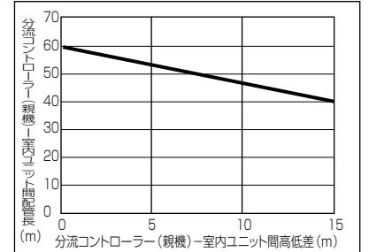
●分流コントローラー - 室内ユニット高低差と枝管長(A)
