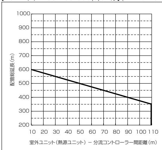
【PURY-(E)P400/450/500(S)CM形】(14/16/18HP)
