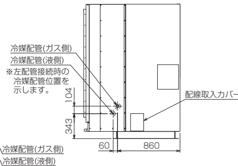
ユニット側面
