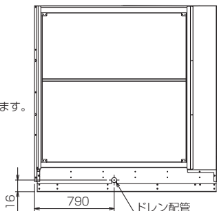
ユニット背面
