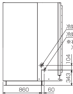
ユニット側面
