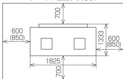
PFAV-P1120・P1400(V) DM-E(1) PFAV-P1250・P1600(V) DM-E(1)-F PFT-P1120・P1400(V) DM-E(1)
