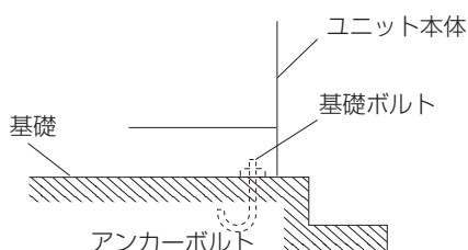
図3 アンカーボルト設置図
