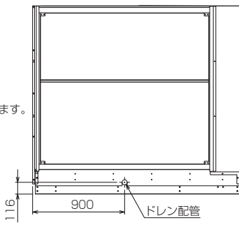
ユニット背面
