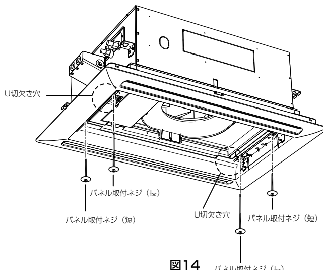
図14 パネル取付ネジ(長)
