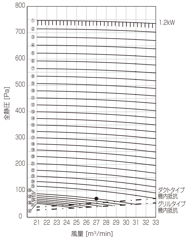
送風機性能線図 PFAV-P80(V)DMJ1
