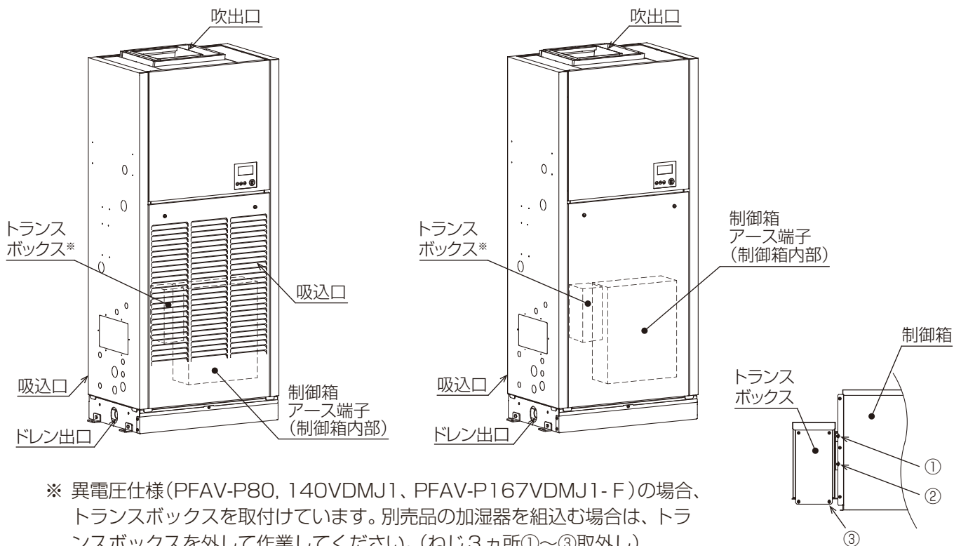
PFAV-P80・140(V)DMJ1の場合
