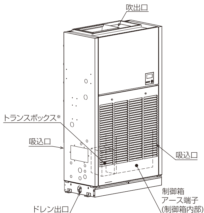
PFAV-P450・560(V)DMJ1の場合
