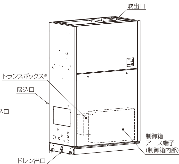
PFAV-P530・670D(V)MJ1-Fの場合
