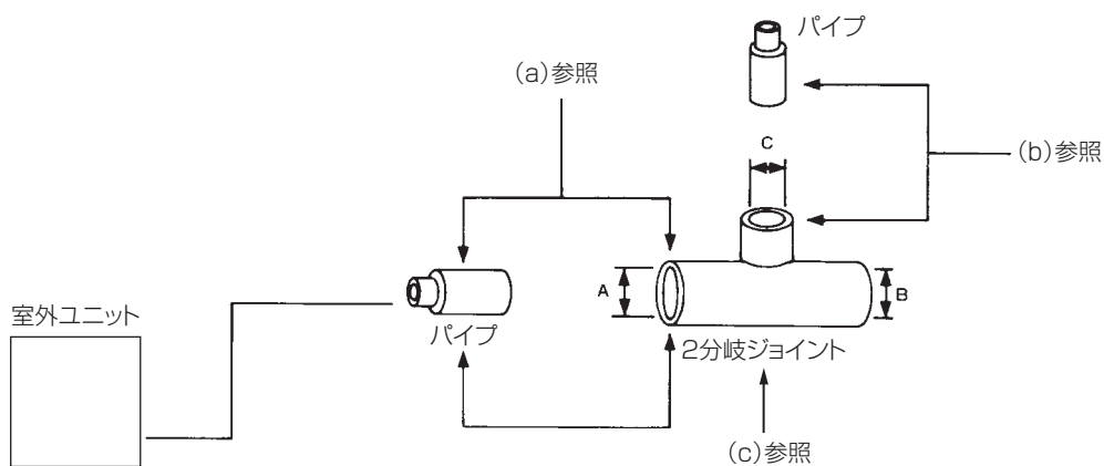
(a) 室外ユニット～分流コントローラー間 (冷媒配管接続例の図-A) の表
