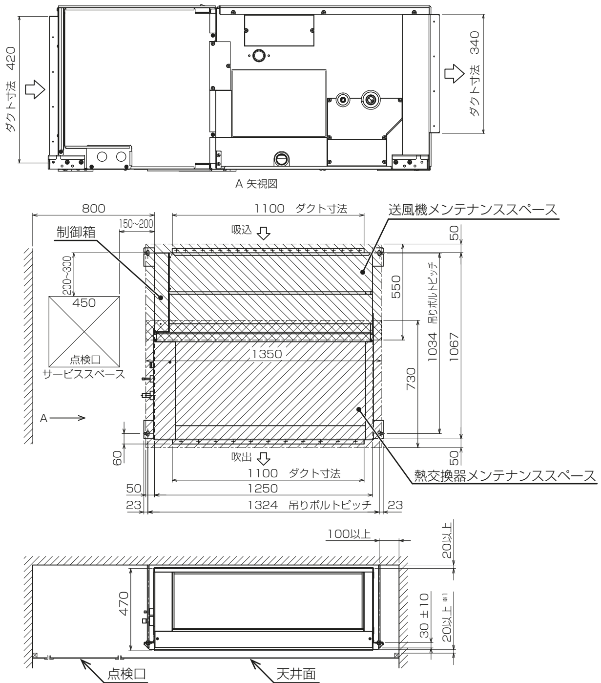
サービススペース詳細図
