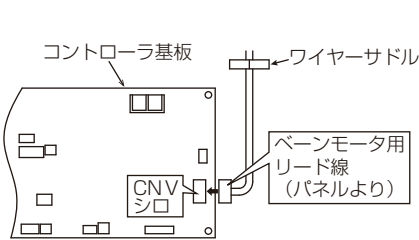
図6-3(c) (PL-RP・LA13以降の場合)
