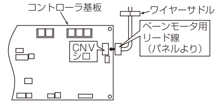
図6-3(a) (PLFY-P・LMG4以降の場合)
