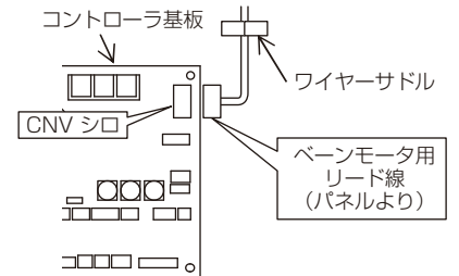
図6-3(b) (PLFY-P・LMG9以降の場合)
