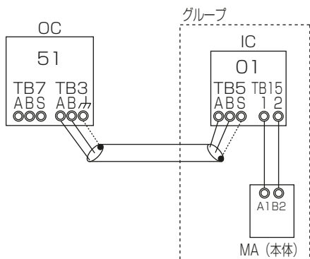
室外ユニット1台の場合
