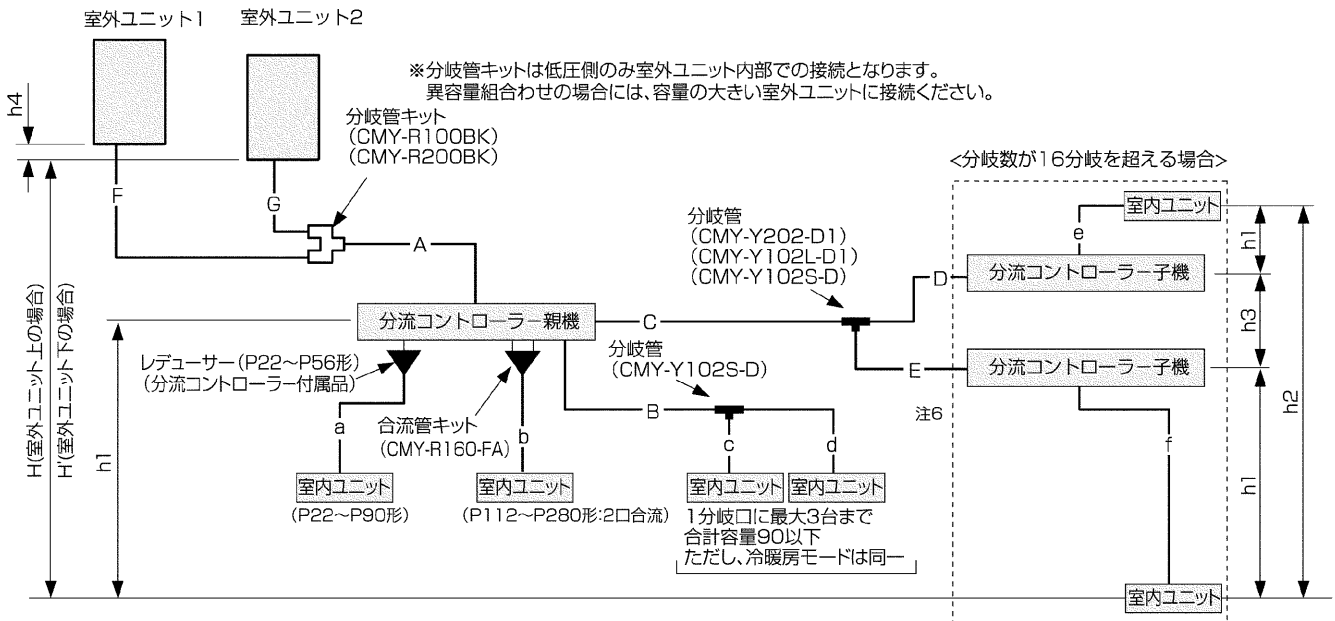
●分流コントローラー - 室内ユニット高低差と枝管長(A)
