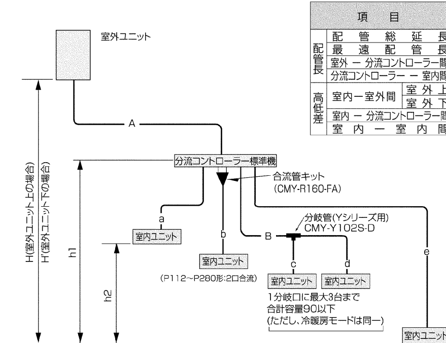
●分流コントローラー - 室内ユニット高低差と枝管長(A)
