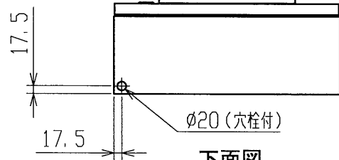
下面図
