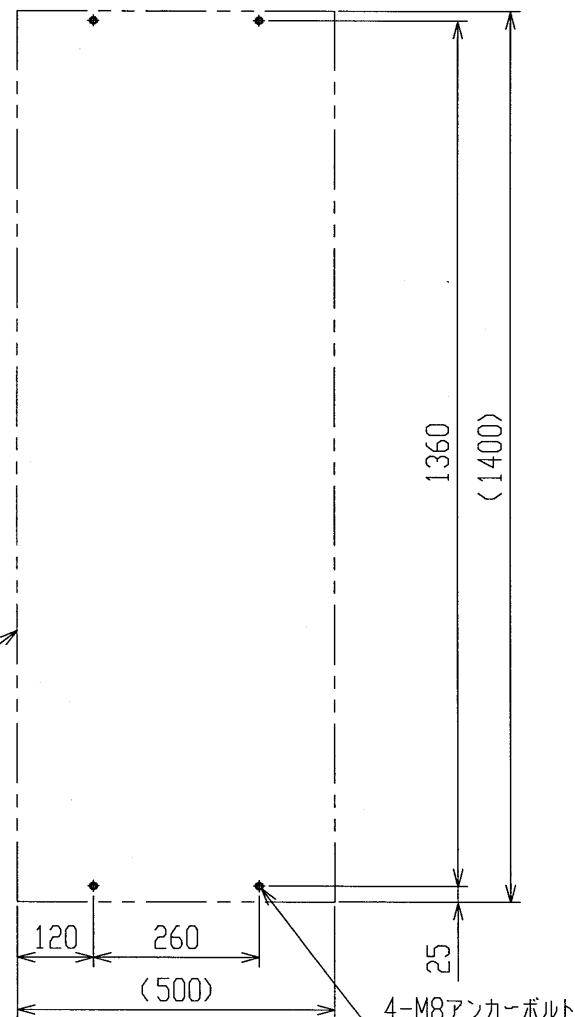
アンカーボルト位置
