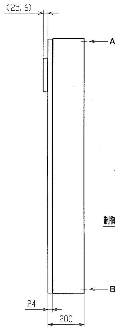
側面図
