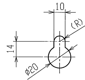
A (上部取付穴)
