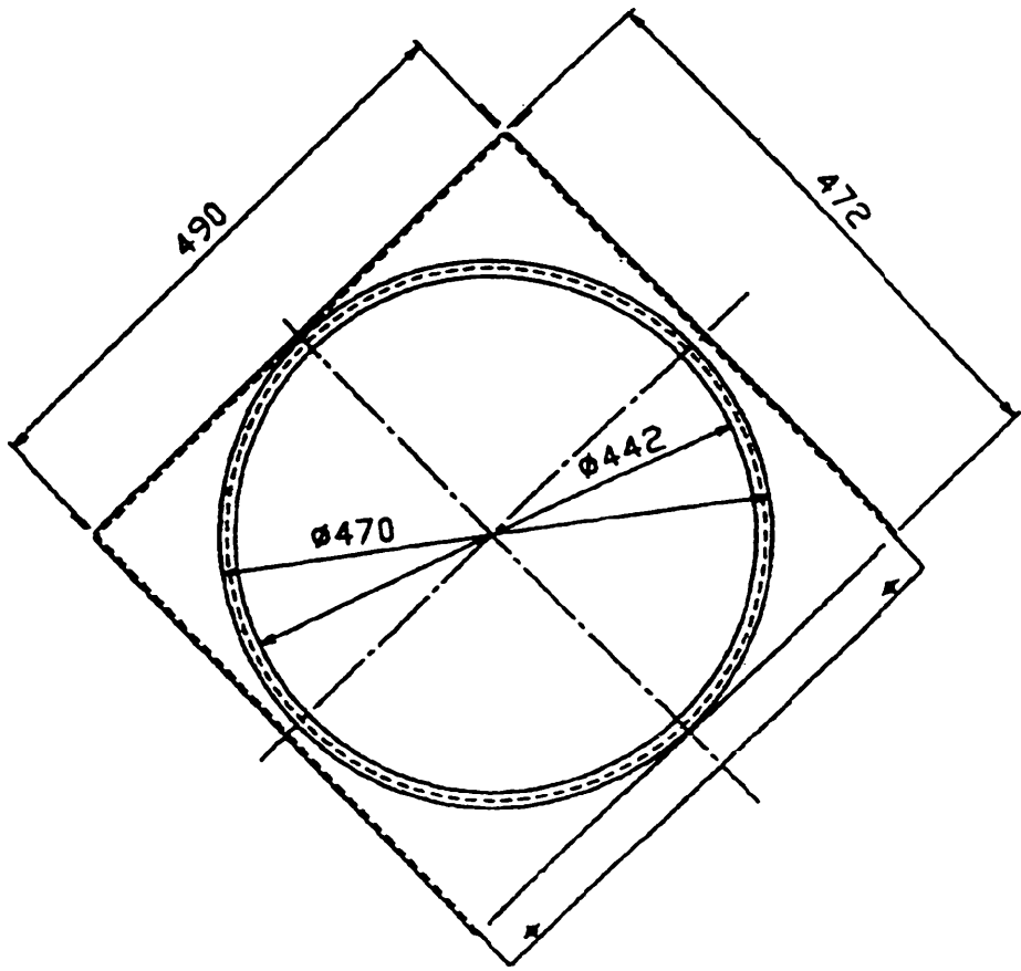
A 矢視
