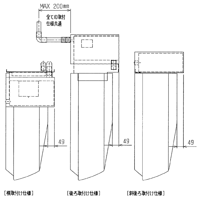
<ドレンアップメカ組込仕様>
