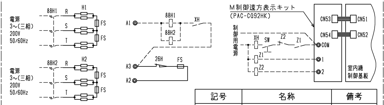
電気ヒーター（再熱用・年間冷房設定時のみ）
