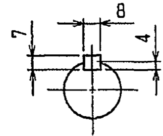
断面A-A
