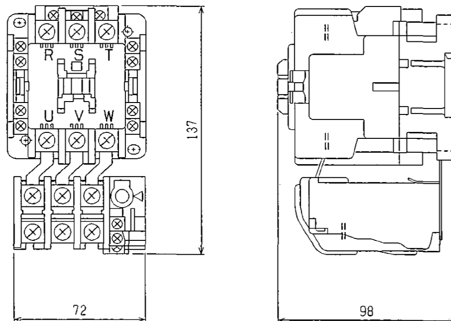
電磁開閉器 PAK-26JTH, PAK-35JTH 戸上電機製 (PAC-CV59~71MPに付属)
