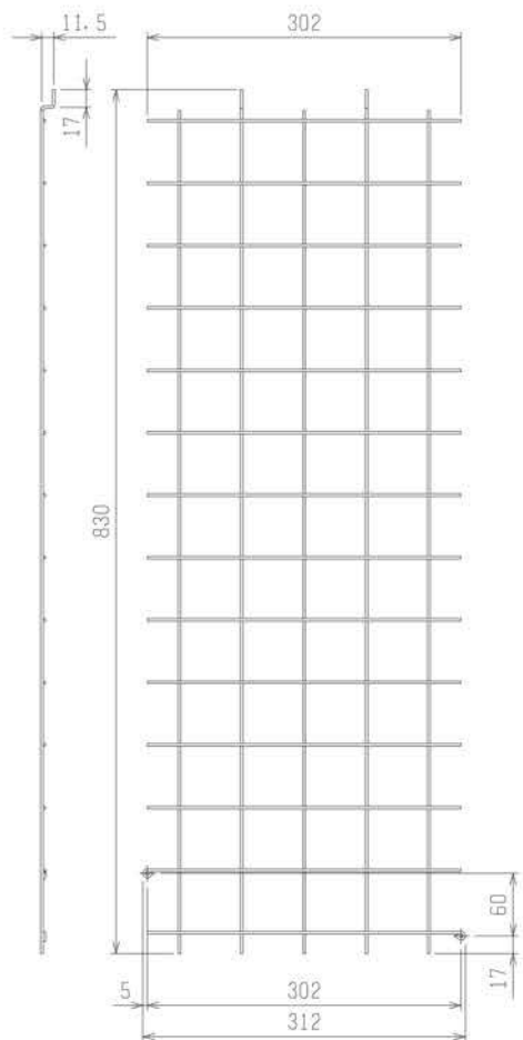
下面防護網 (A-左)
