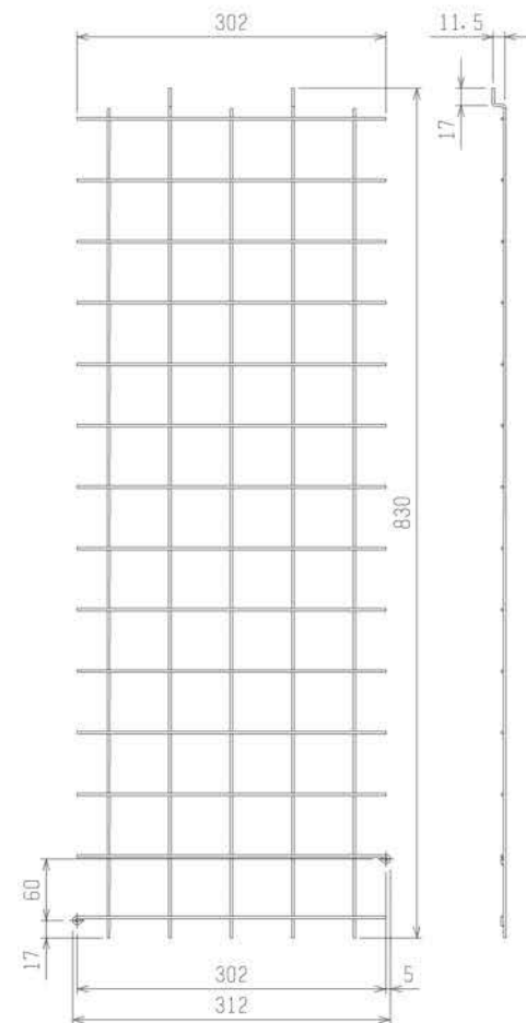
下面防護網 (A-右)
