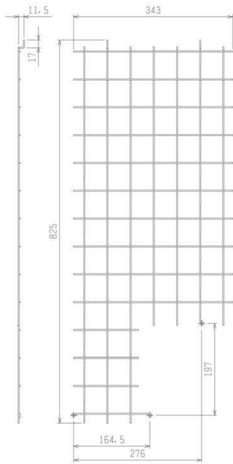
下面防護網 (B-左)
