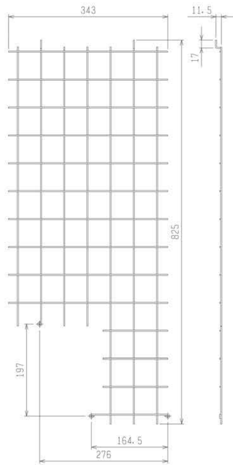
下面防護網 (B-右)
