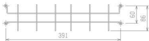
下面防護網 (中央)
