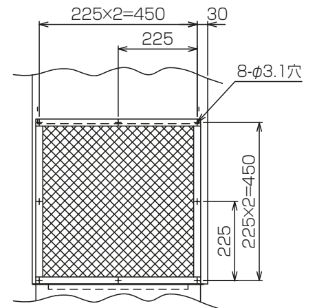
吸込口詳細図(金網ありの場合)
