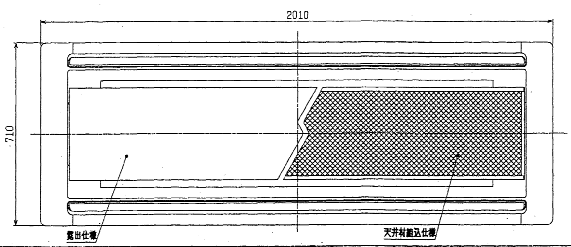
フィルタ外形図
