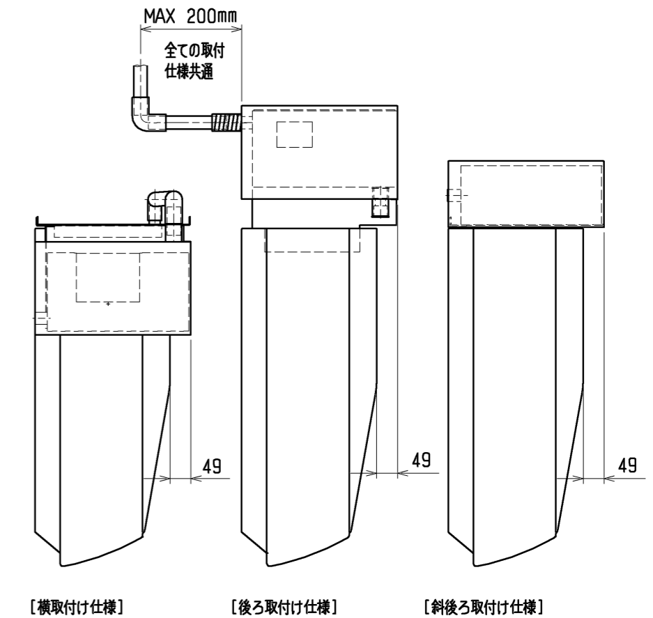
<ドレンアップメカ組込仕様>
