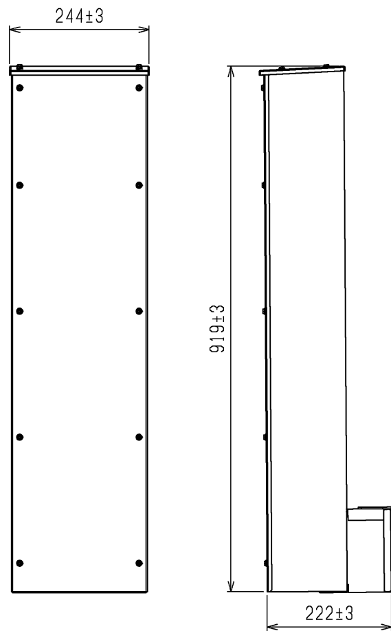
防雪ダクト外形図
