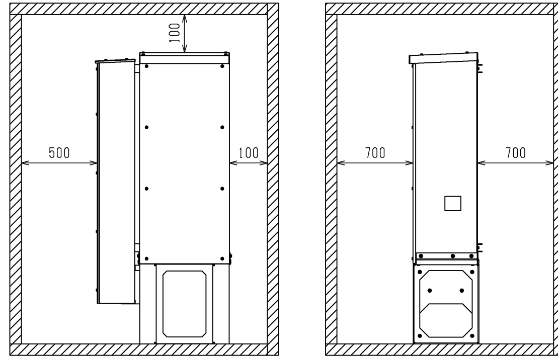
保守・排熱スペース 注2
