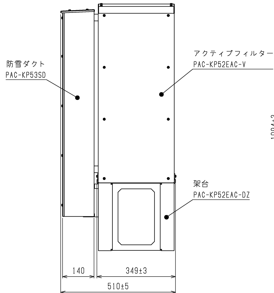
防雪ダクト外形図
