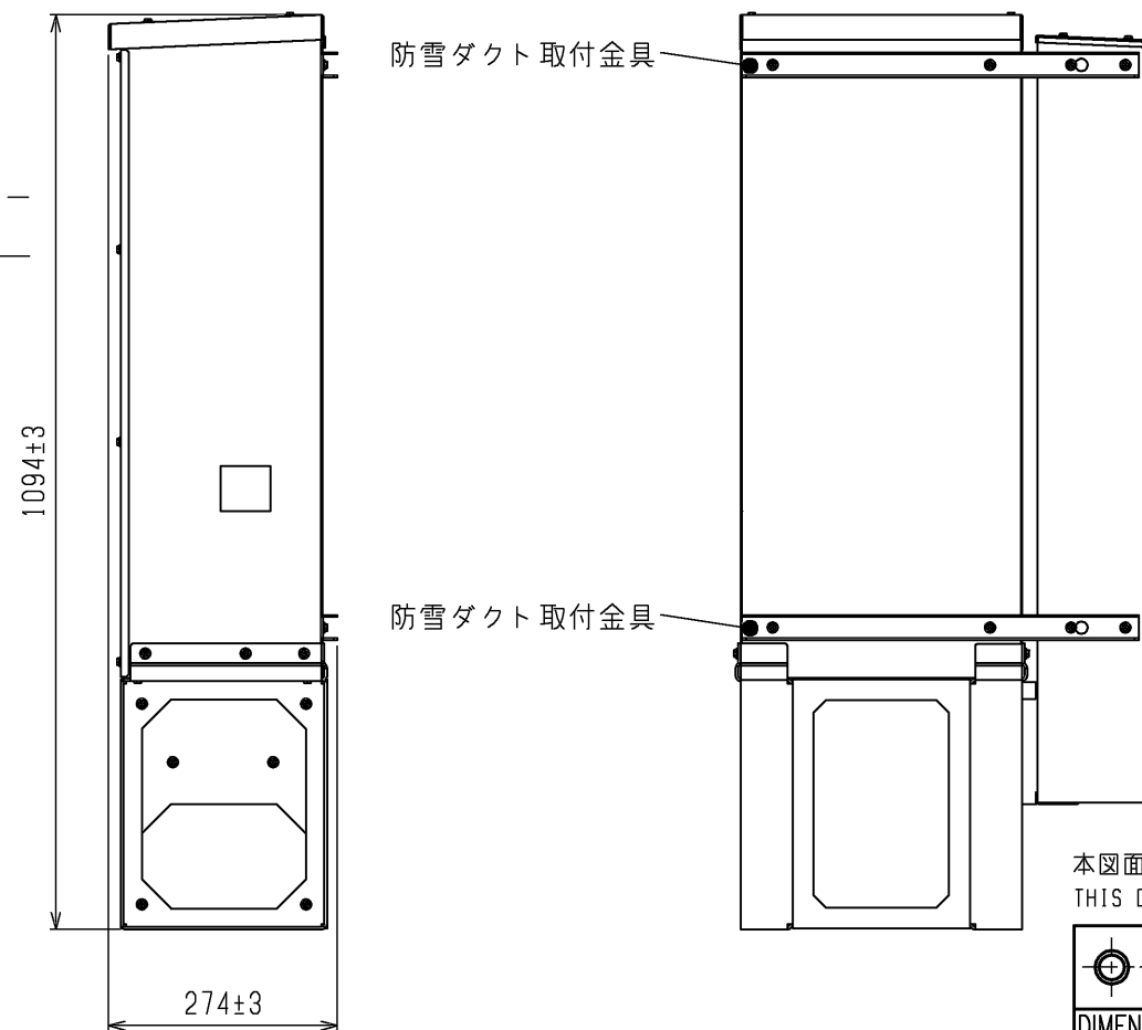
アクティブフィルターへの取付図
