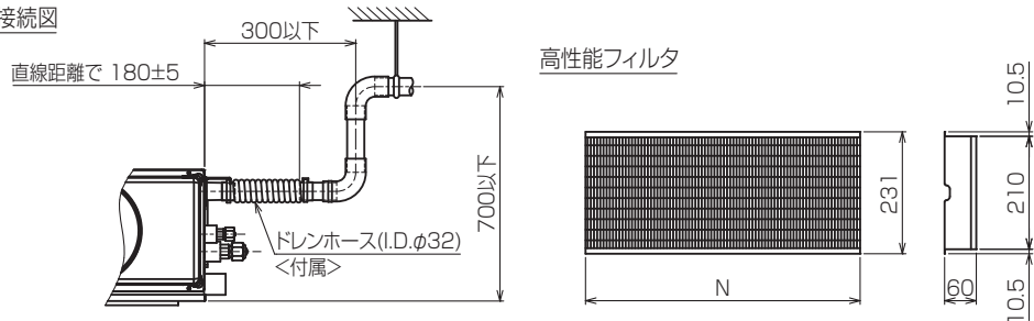
ドレン配管接続図
