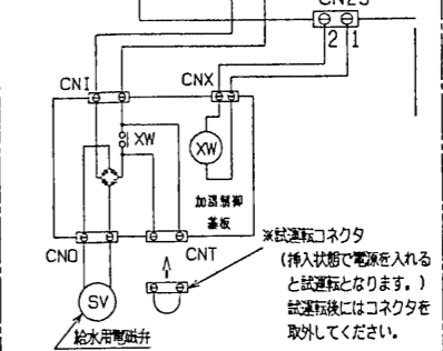
配線図
