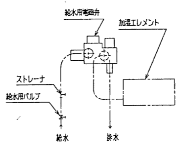
接続図
