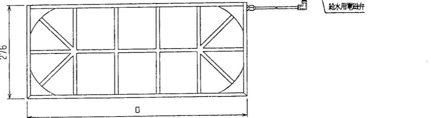
加湿エレメント外形図
