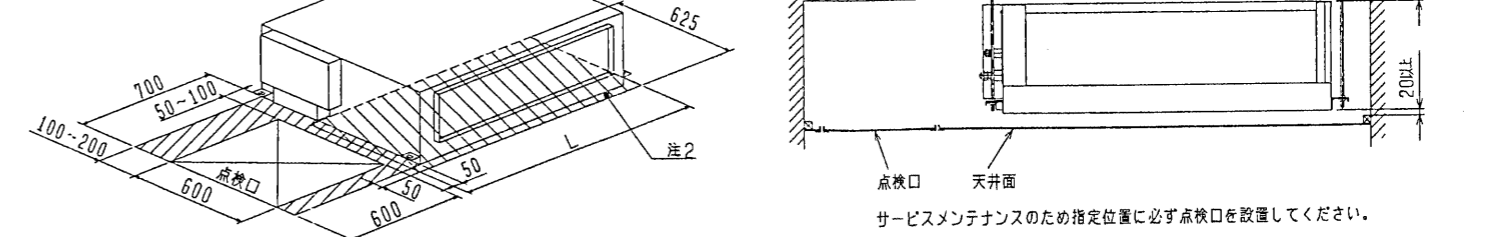
サービススペース詳細図
