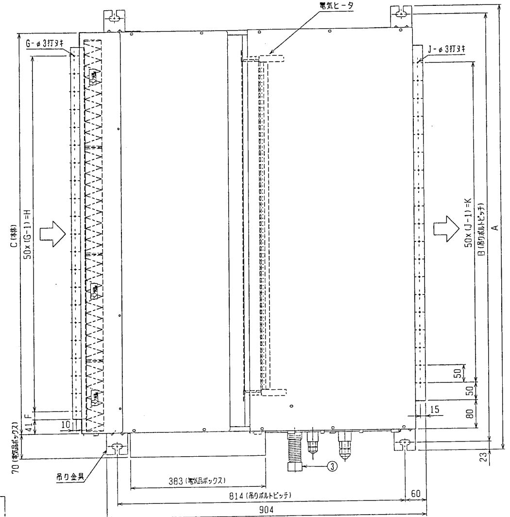
電気ヒータ外形図
