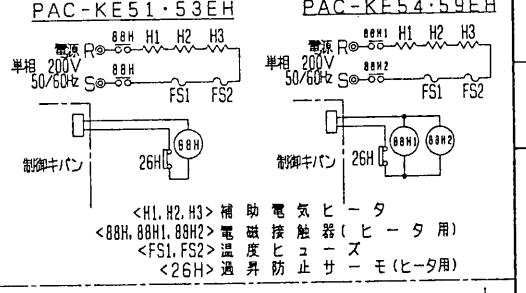
配線図
