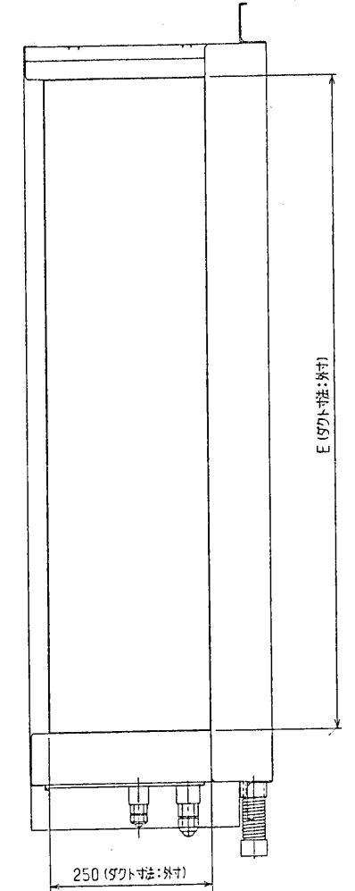
電気ヒータ外形図
