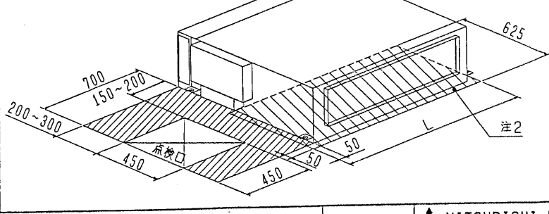
ヒータ+ロングライフフィルタ組込み
