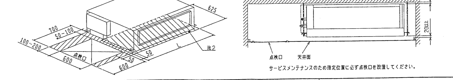
サービススペース詳細図
