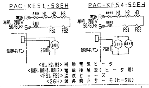
配線図
