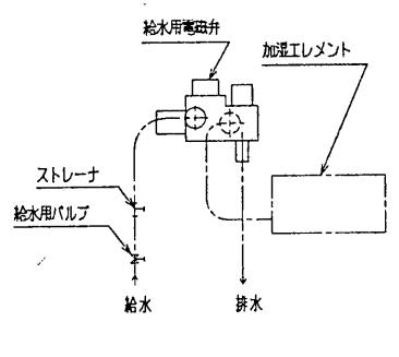
接続図
