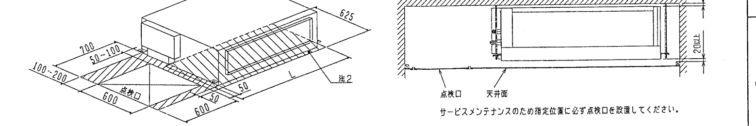
サービススペース詳細図
