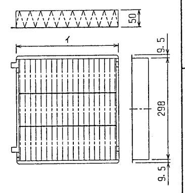
ロングライフフィルタ外形図
