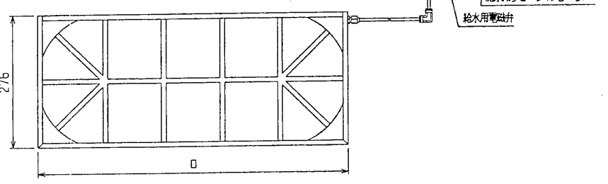
加湿エレメント外形図
