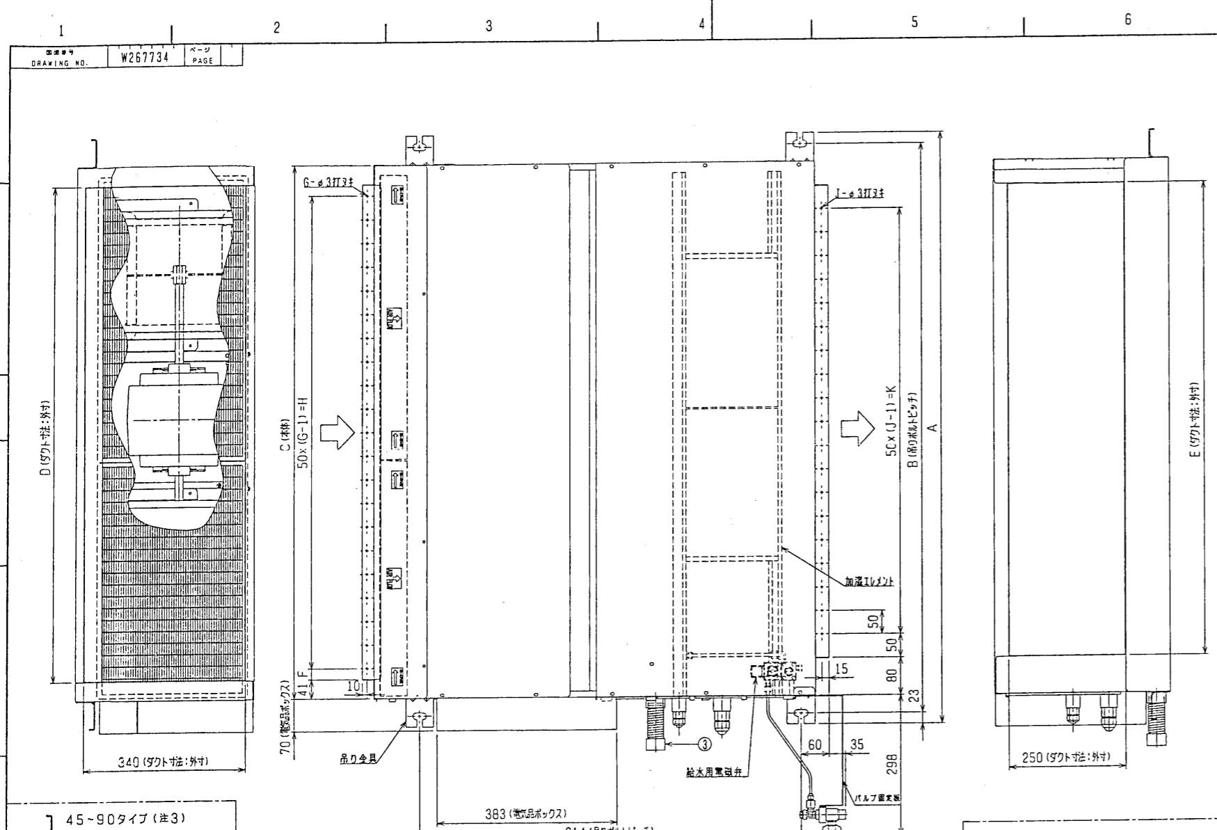
加湿エレメント外形図
