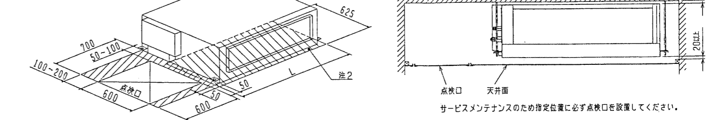
サービススペース詳細図
