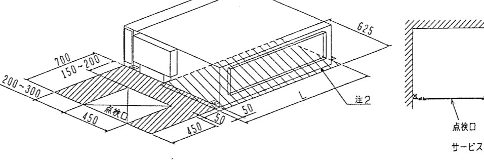
サービススペース詳細図
