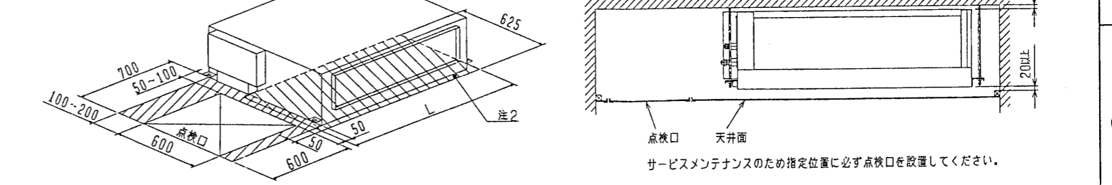
サービススペース詳細図 (Service Space Detail Diagram)
