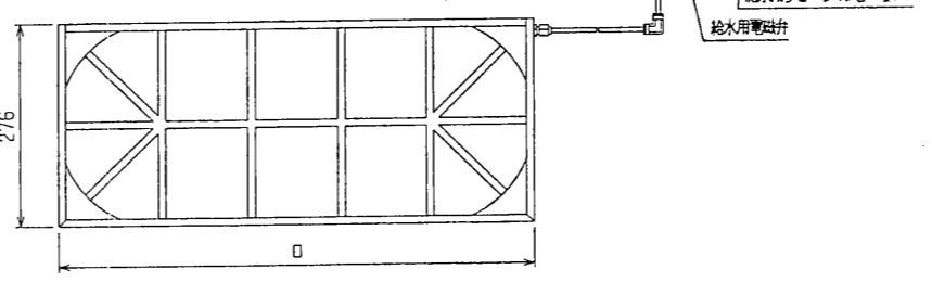
加湿エレメント外形図 (Humidifier Element External View)
