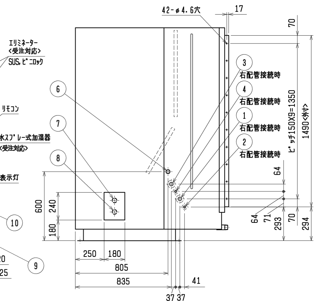
水スプレー式加湿器組込
