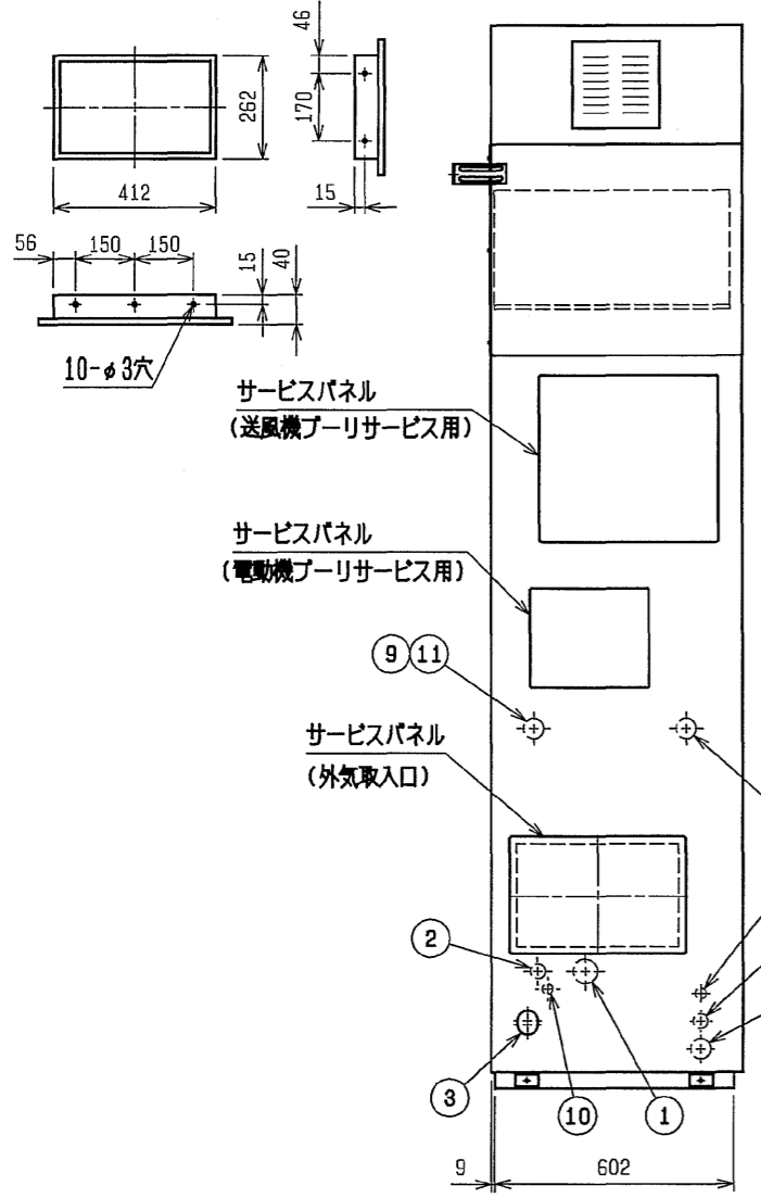
外気取入フランジ<別売部品> (Outdoor Air Intake Flange <Optional Part>)
