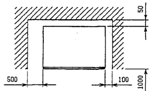
通風・サーヒースペース 通常最低必要寸法を示します。
