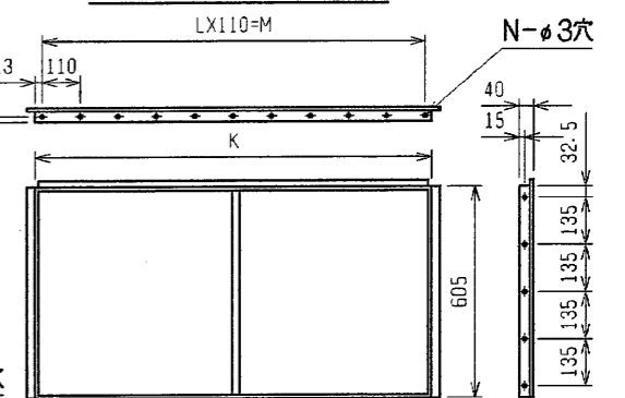
後吸込ダクトフランジ
