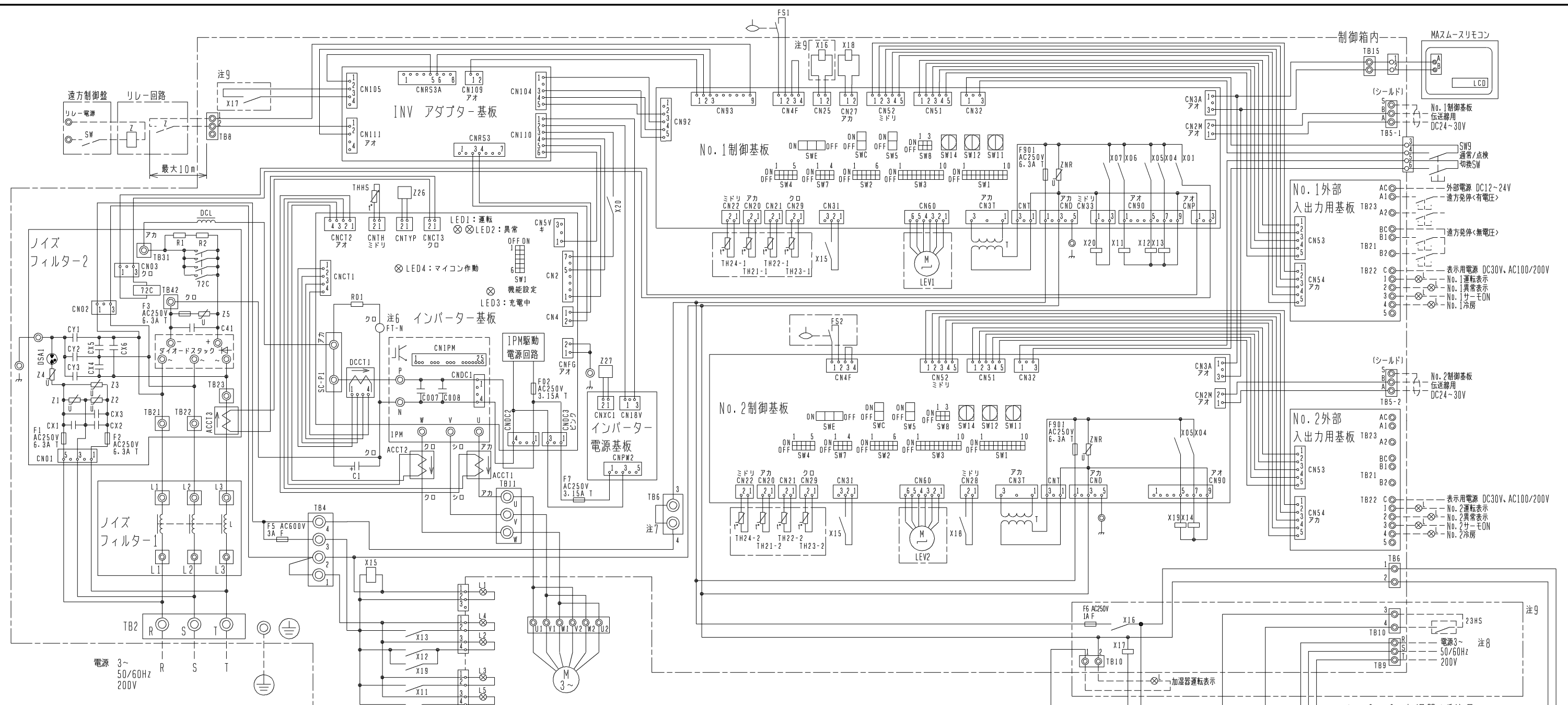
記号説明
