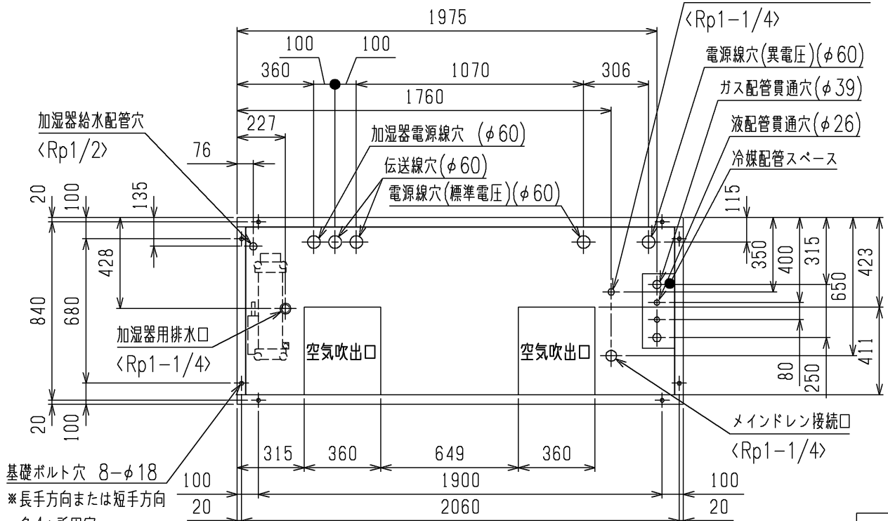
床面寸法図
