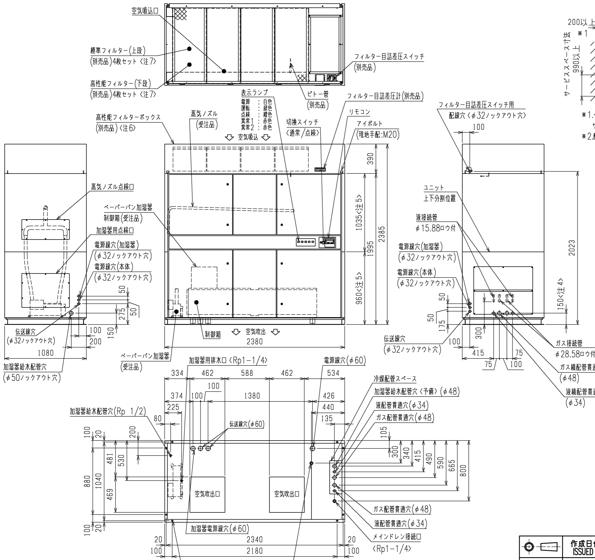
床面寸法図
