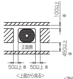
<単位:mm>
