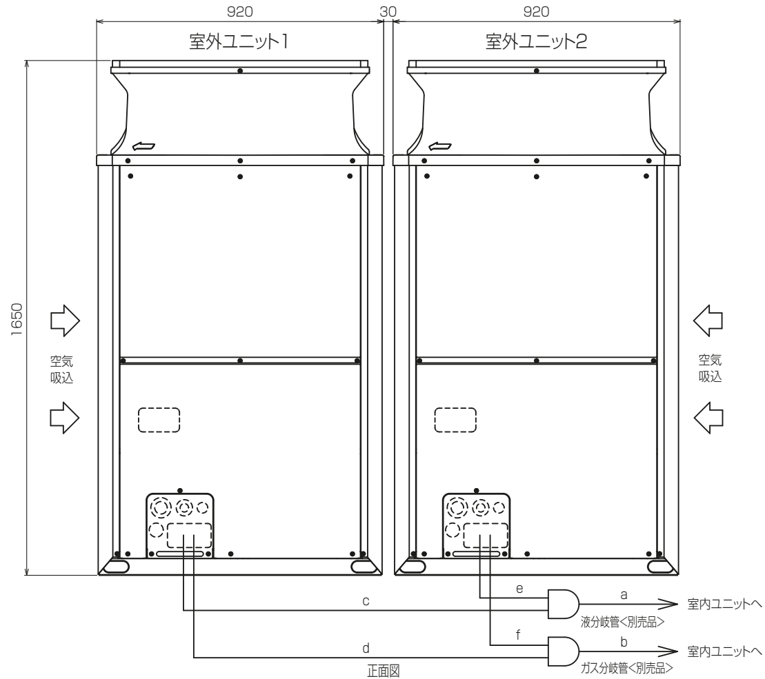
正面図
