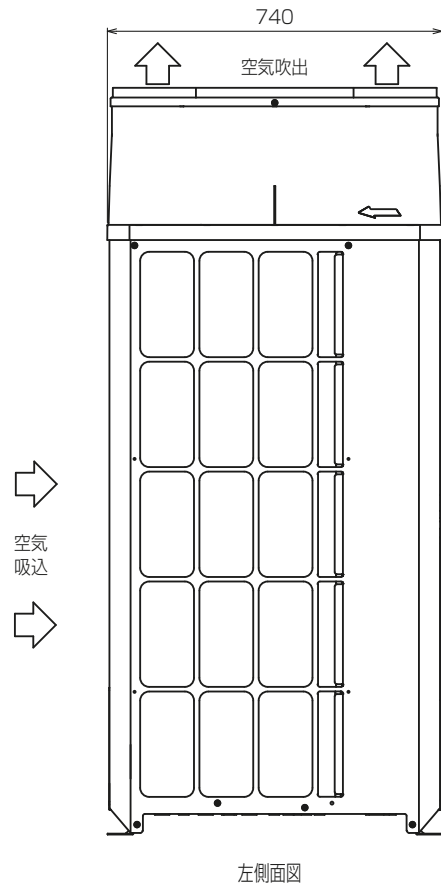
左側面図
