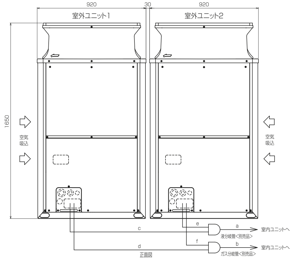
正面図
