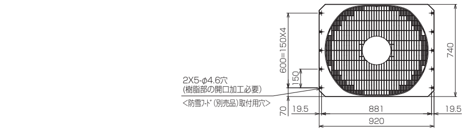
接続管仕様
