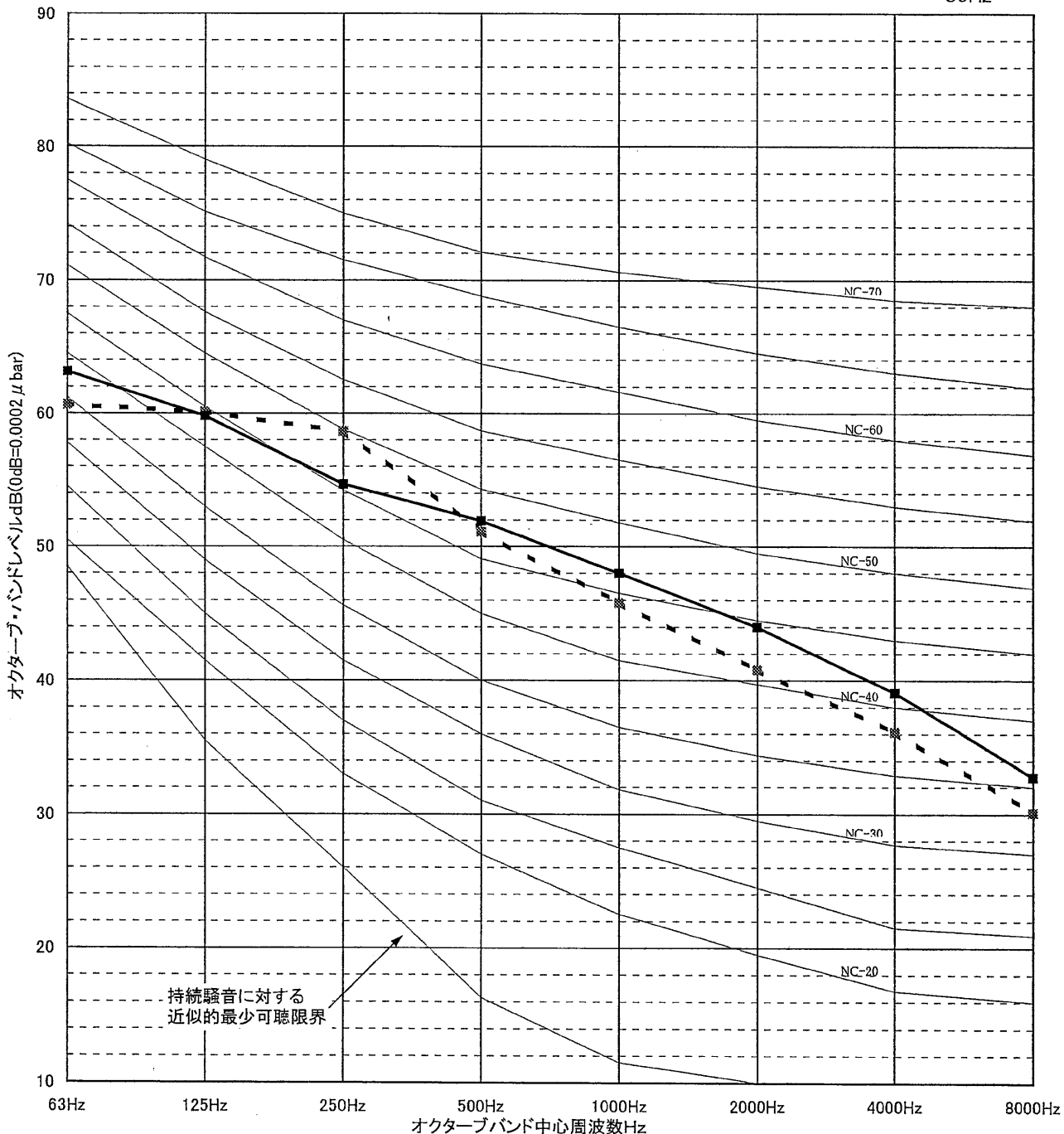
騒音レベルのオクターブ値
