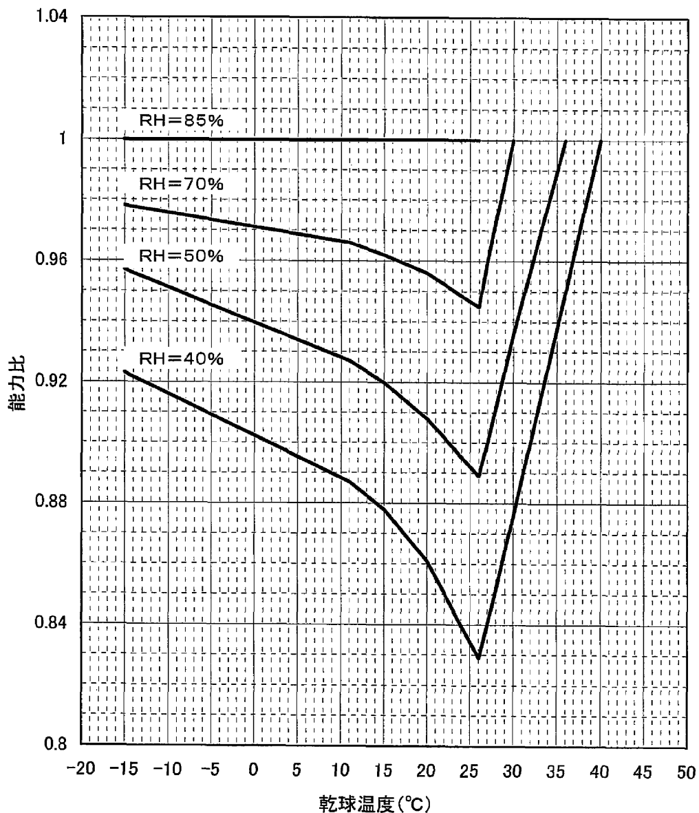
加熱能力相対湿度補正線図(50/60Hz)
